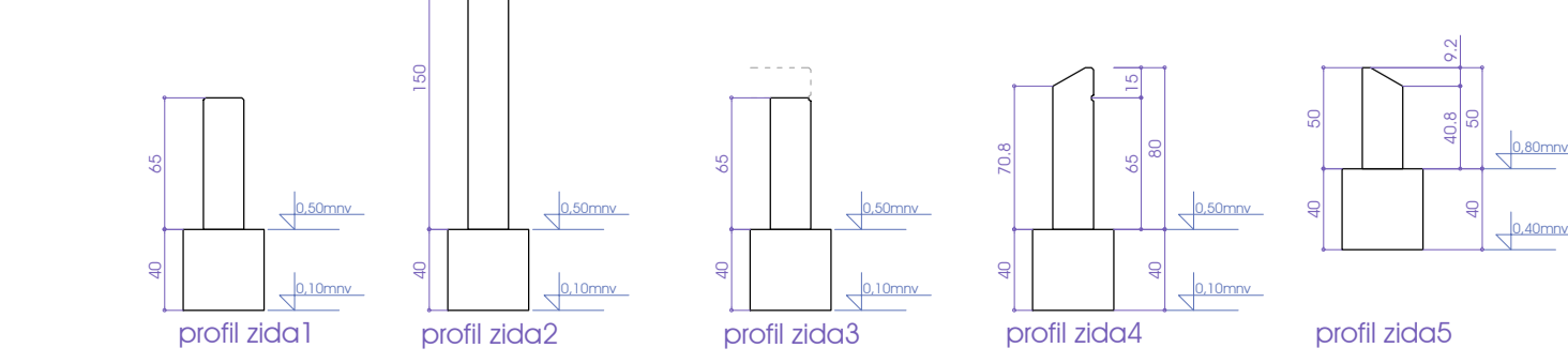
DETALJ - TIPOVI ZIDIĆA SUNČALIŠTA
