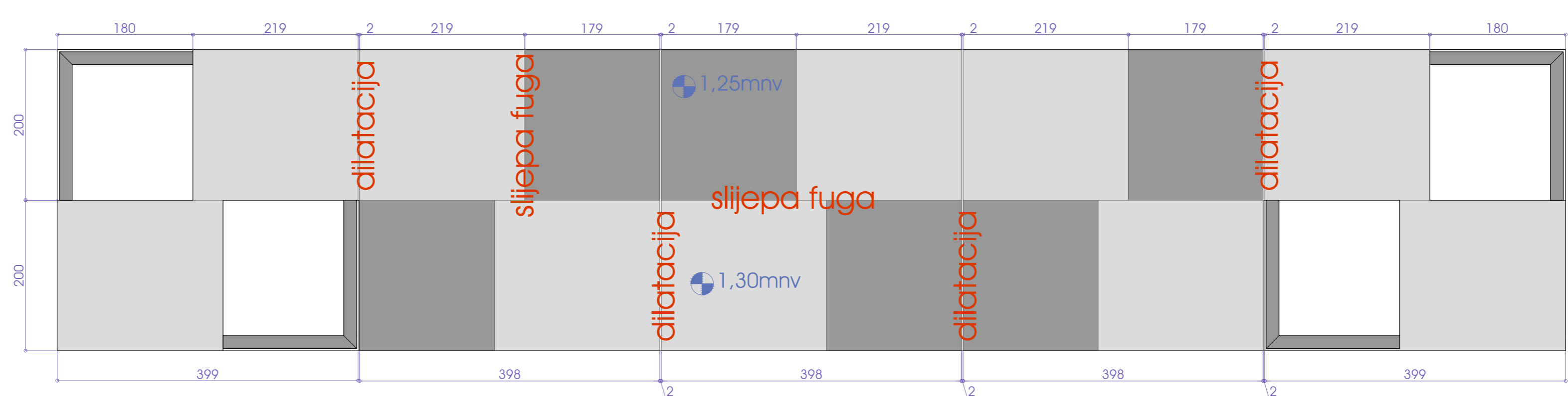
TLOCRT HORIZONTALNIH PLOHA OD DEKORATIVNOG BETONA
